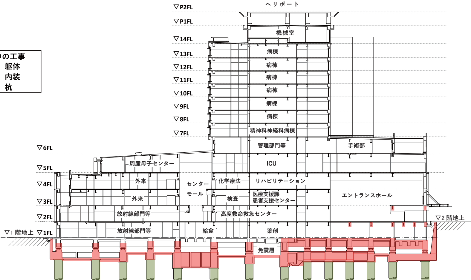
断面図
