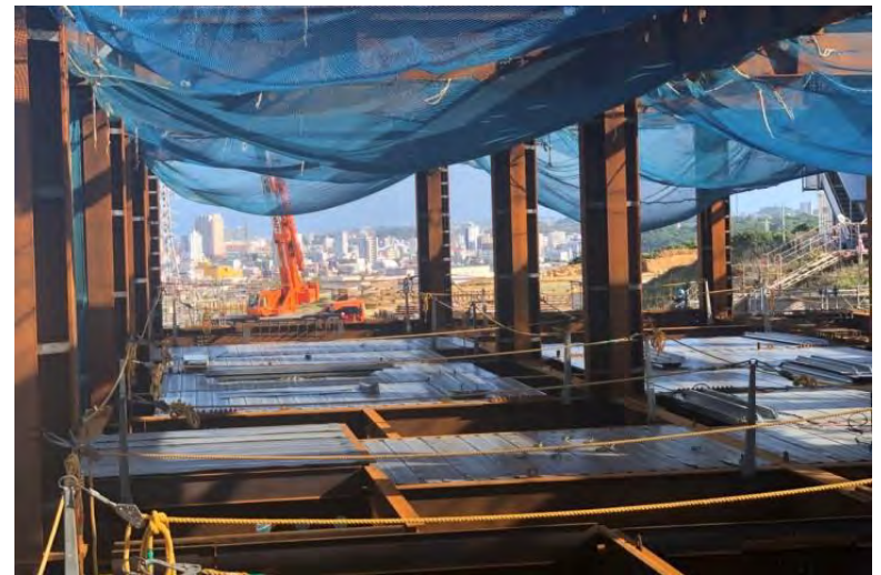
写真⑫ (鉄骨工事 2階 床デッキ施工状況)
