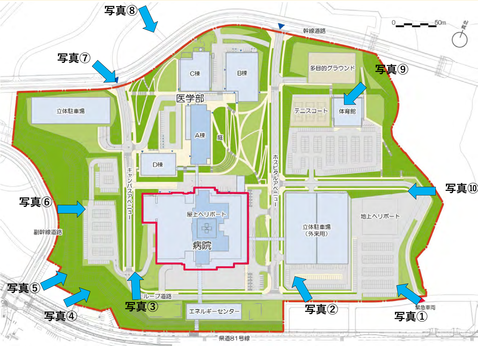
配置図
