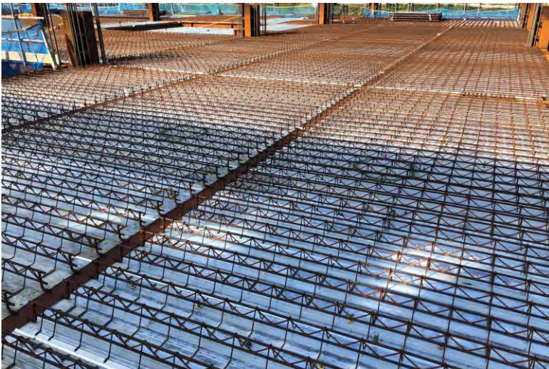
写真⑪ (型枠工事 4階 デッキスラブ施工状況)
