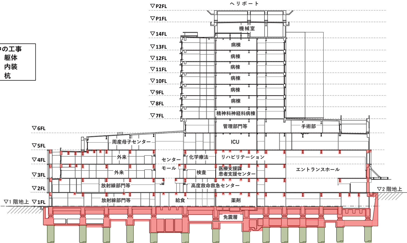
断面図
