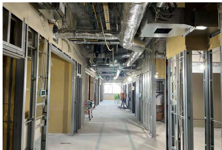
写真⑫ (内装工事 8階病棟 廊下施工状況)
