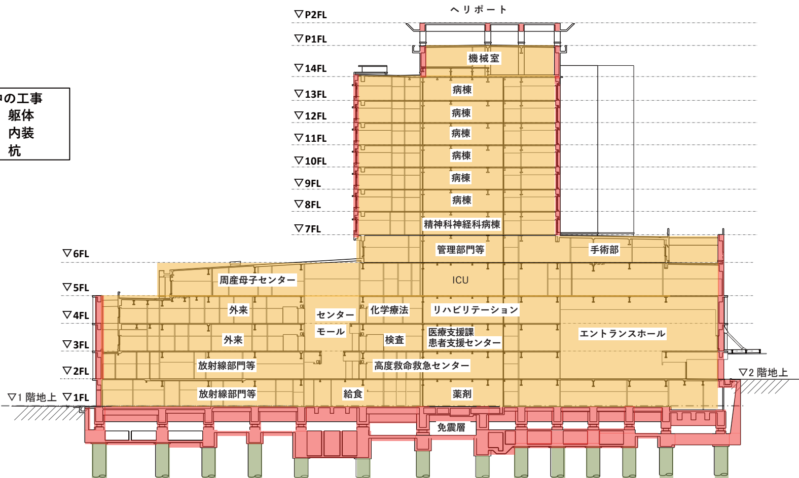
断面図
