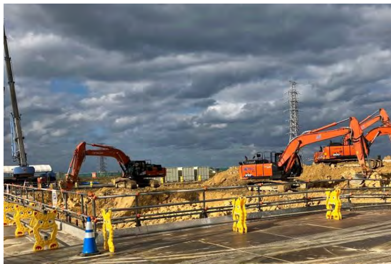
写真⑫ (土工事 C棟 掘削状況)
