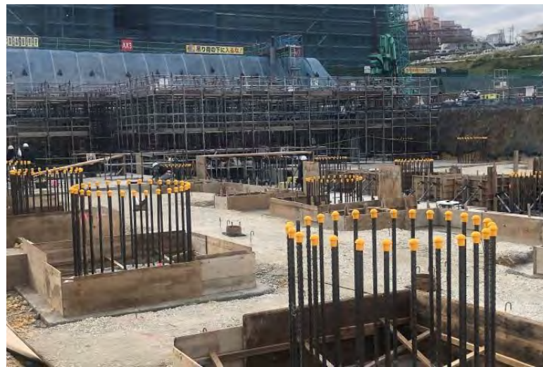
写真⑩ (躯体工事 A棟 レベルコンクリート打設前)
